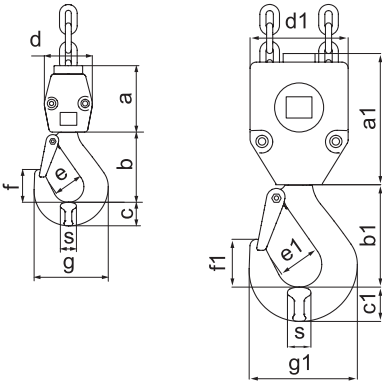
Крюковая подвеска CLF 1/1
